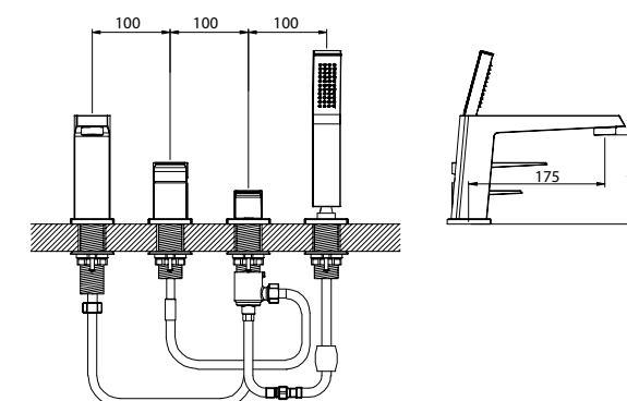
ARL-VIM4-CRM Смеситель для ванны однорычажный с ручным душем
