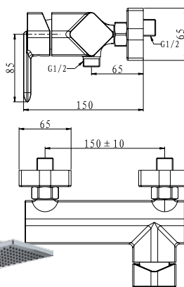
CRY-ESDM-CRM Смеситель для душа
