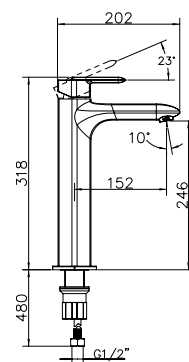
CRY-LMC-CRM Смеситель для накладных раковин
