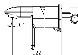
CRY-BCM-CRM Встраиваемый смеситель для раковины
