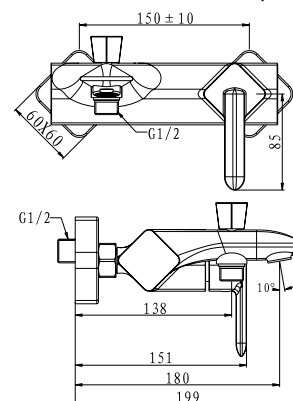
CRY-VASM-CRM Смеситель для ванны и душа
